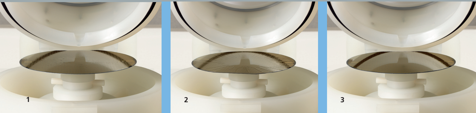
1–3 Beschichten eines prozessierten Wafers mit einem vorapplizierbaren Klebstoff mittels Spin-coating.
