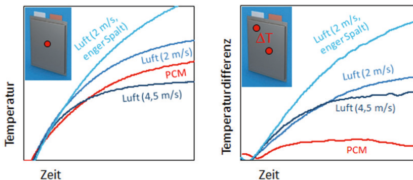
Abb. 1 Kerntemperatur und Temperaturdifferenz in einer Zelle bei einer Schnellladung bei verschiedenen Temperierkonzepten
